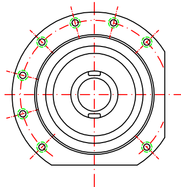
ВИД СО СТОРОНЫ А
