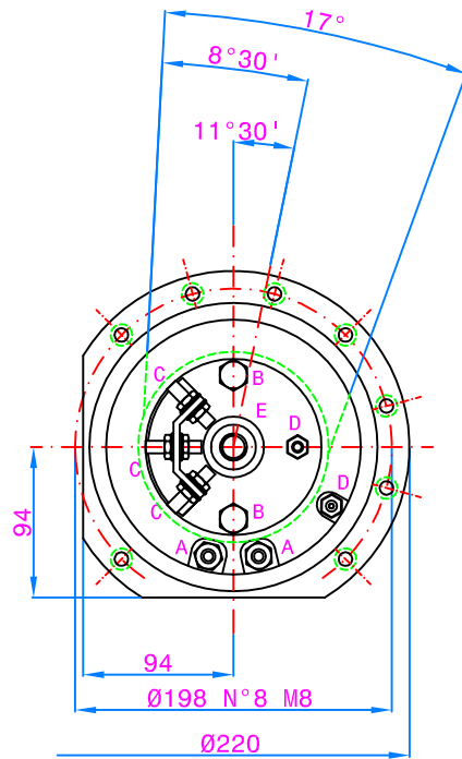
ВИД СО СТОРОНЫ В
