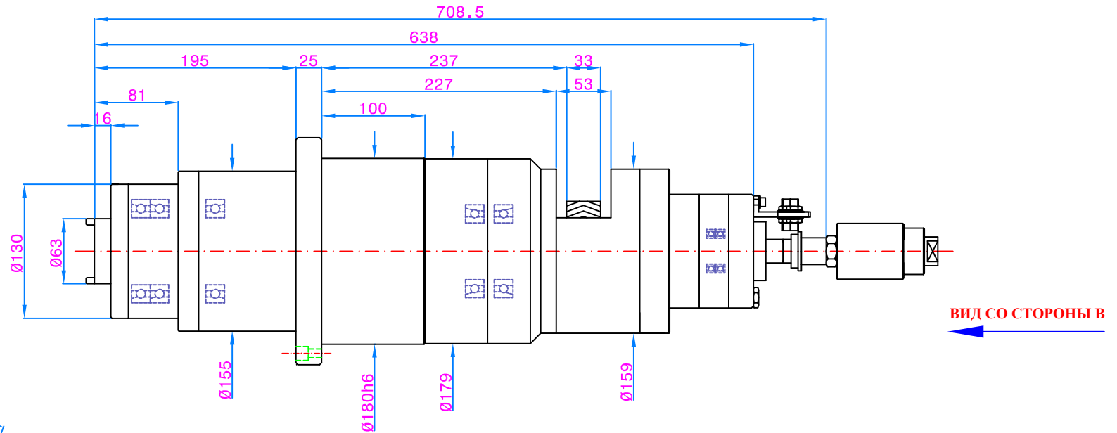
ВИД СО СТОРОНЫ А
