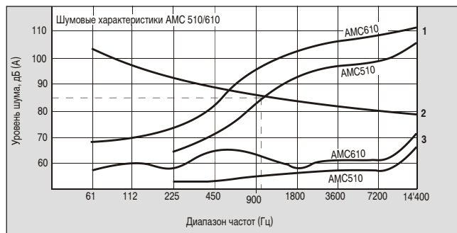
1 - без фильтра-пневмоглушителя 2 - SUVA-кривая предельно допустимого уровня шума 3 - с фильтром-пневмоглушителем
